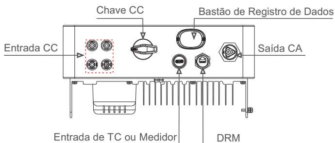
Figura 1.2 Vista inferior
