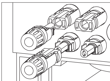
Figura 4.12 Conectar ao Inversor
